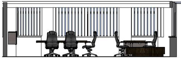
WIDOK A. 1:50
